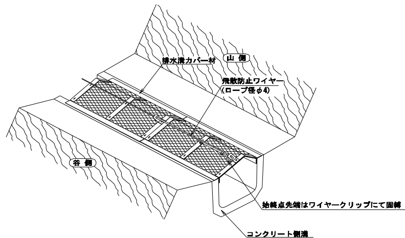
飛散防止用ワイヤー取付状態図
